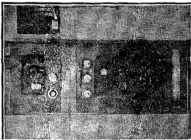
El amplificador de potencia con 6 válvulas e instrumento de control.
