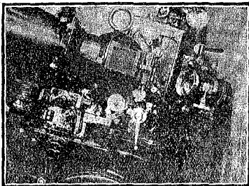
Detalle de la parte principal de uno de los dos proyectores. A la extrema derecha se distingue la lente objetiva de 104 milímetros de diámetro.
