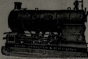
MAQUINA SEMIPERMANENTE PARA LUZ ELECTRICA.
